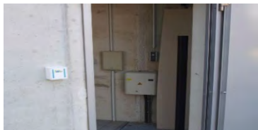
DAKO-TS „Basis“ mit schwarzem Säulenlichtschrankenempfänger
